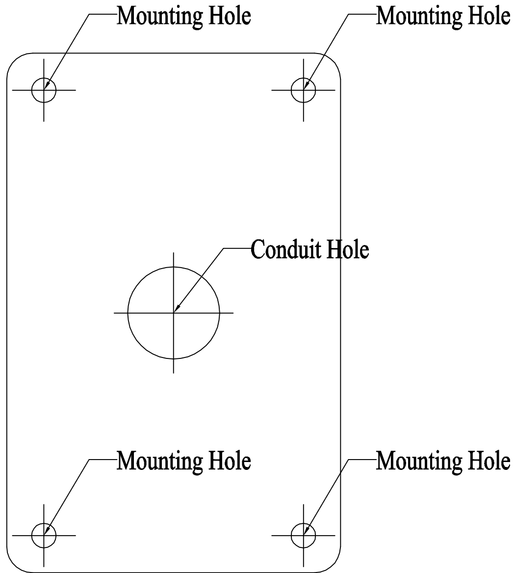
Drill template(scale 1:1)
