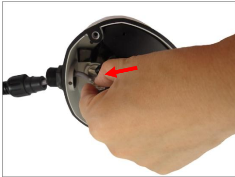
Using Flex Conduit
